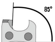
横刃の目立て角度
