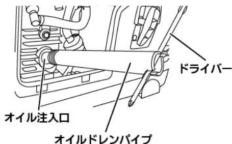
オイルドレンパイプ
