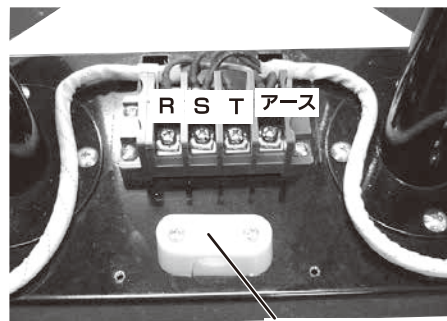
電源コード固定具
