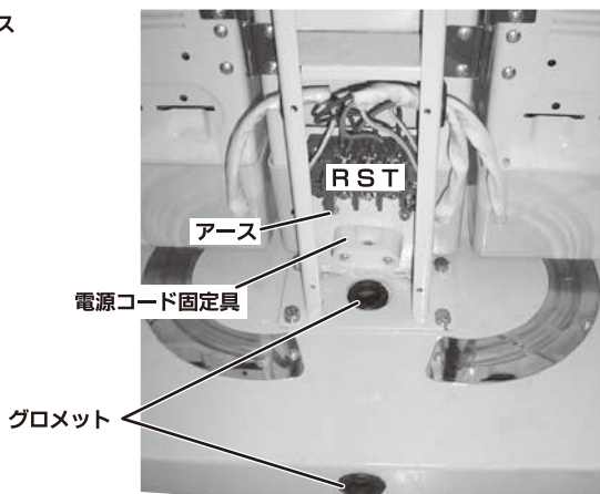
電源コード固定具
