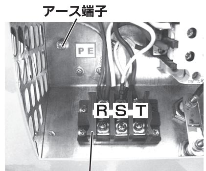
アース端子 端子台
