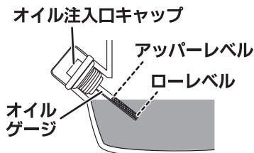
オイル注入口キャップ
