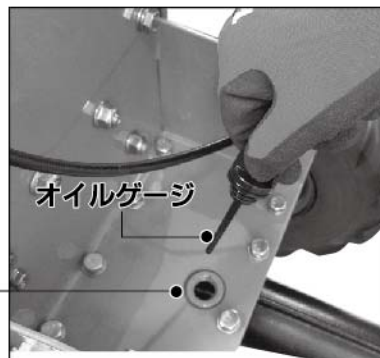
ギヤオイル注入口
